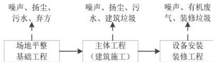
图 4 项目施工期工艺流程及产污环节图
