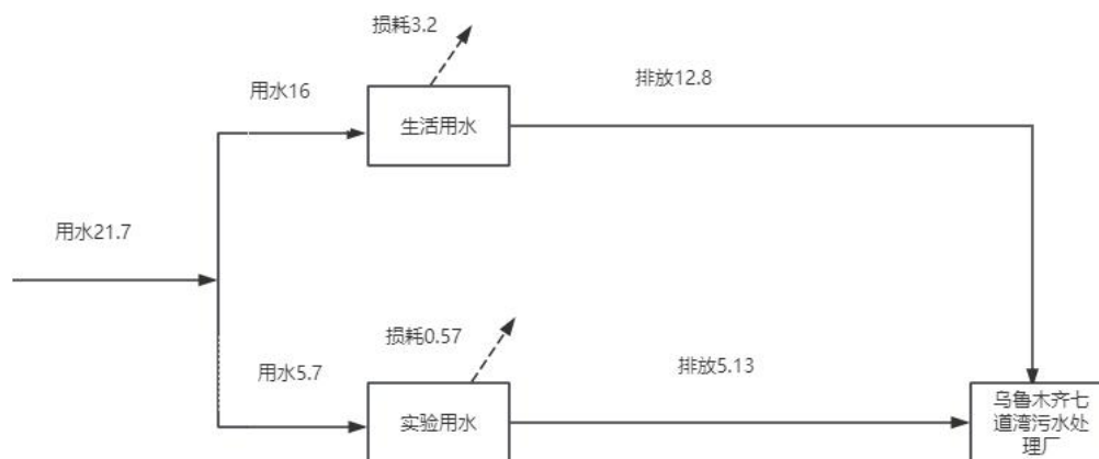
图 1 项目水平衡图 单位：立方米/年
