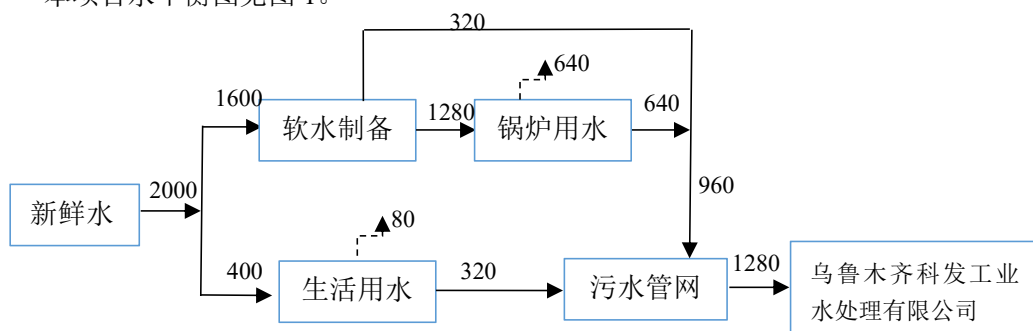
图 1 本项目水平衡图 单位：立方米/年
