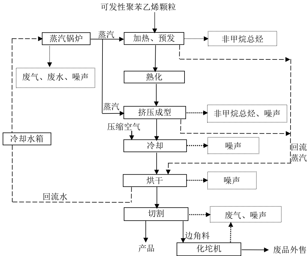
图3 改性模塑保温板生产工艺流程及产排污环节图
