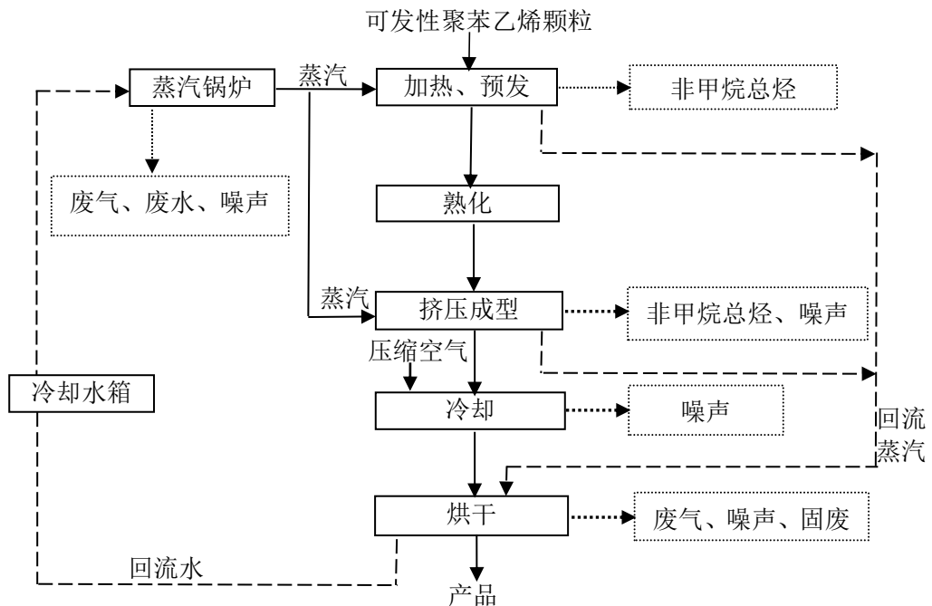
图 4 节能保温中转箱生产工艺流程及产排污环节图
