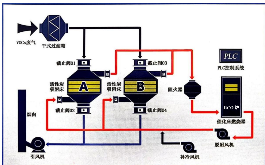
图 5 蓄热式催化燃烧设备（RCO 一体化装置）处理工艺流程图
