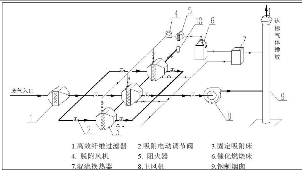
图 10 催化燃烧脱附工艺流程图
