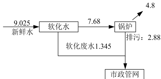
图 5 本项目锅炉系统给、排水平衡图（单位 吨/小时）
