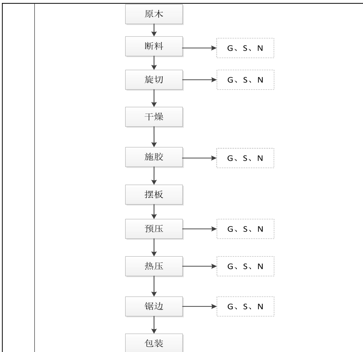
图8 细木板和多层板生产工艺流程及产污环节图
